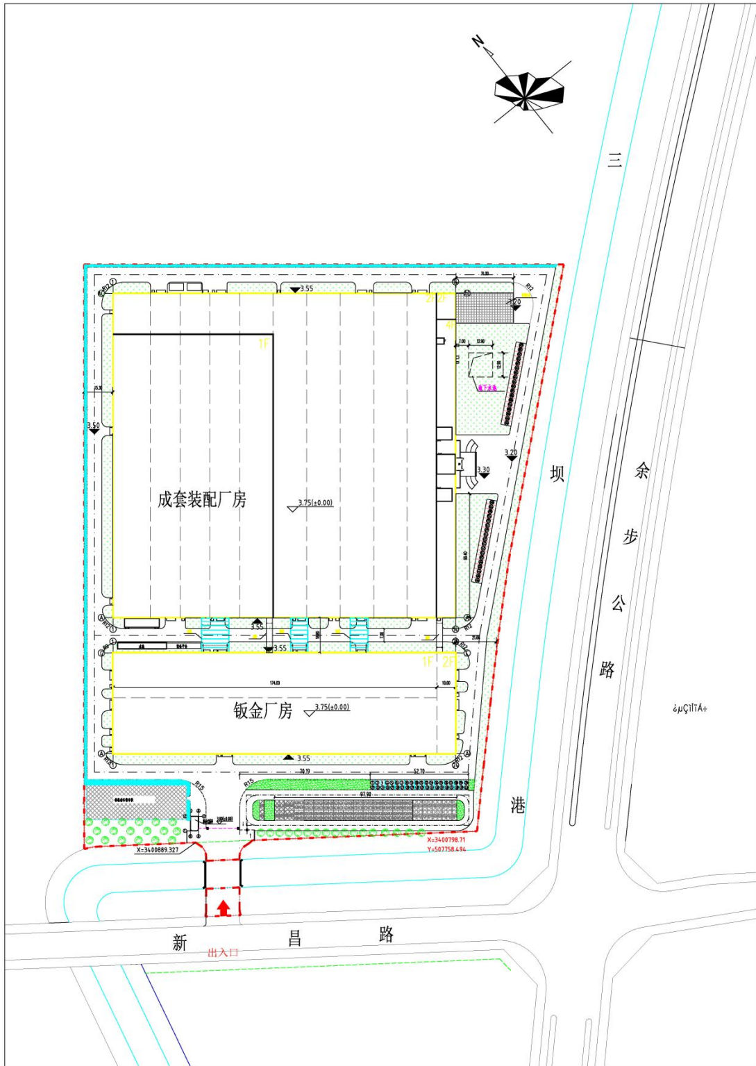
图 3-7 华东园区厂区平面图
