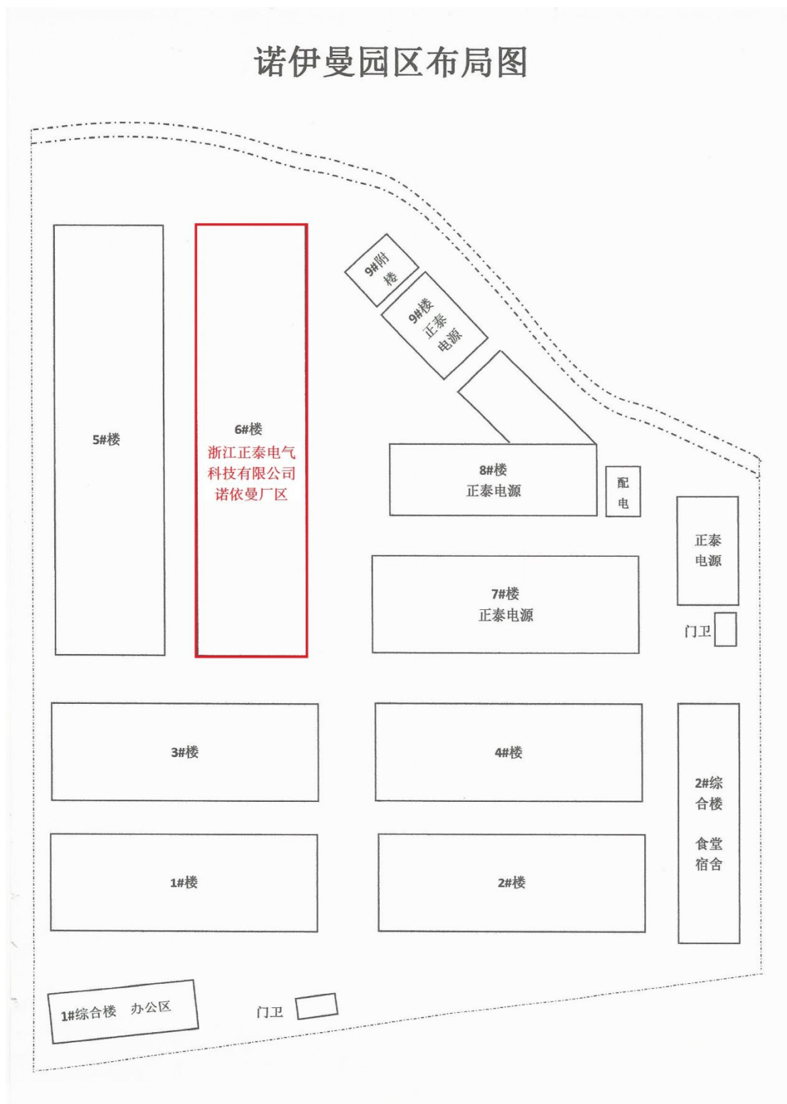
图 3-6 诺依曼厂区平面图
