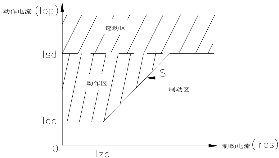
图 5 比率差动保护动作特性图
