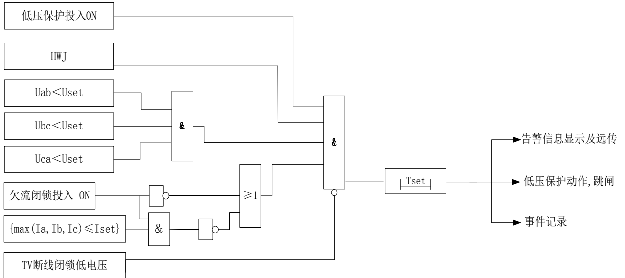
图 16 低压保护动作逻辑图
