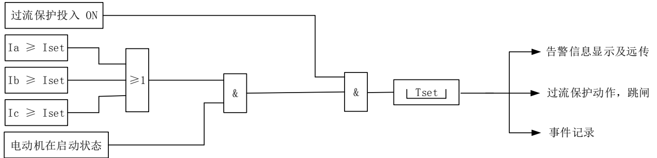
图 10 一段保护逻辑框图
