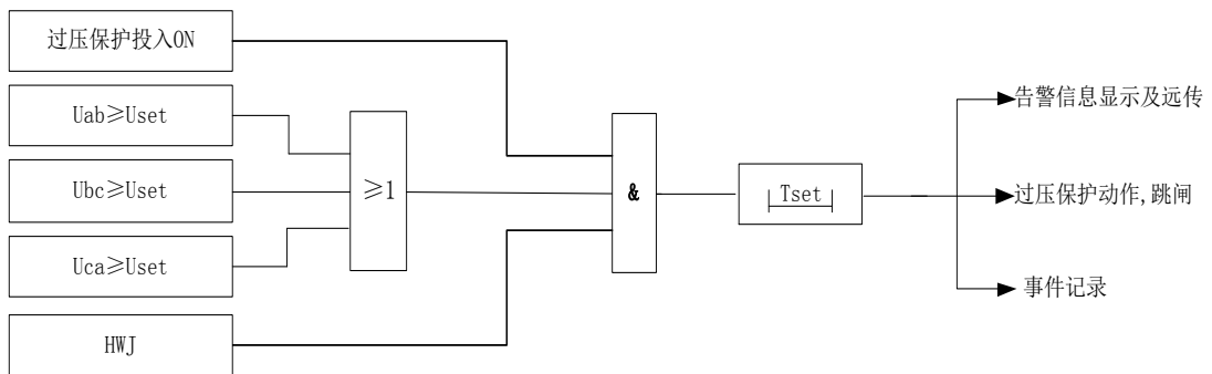
图 17 过压保护动作逻辑图
