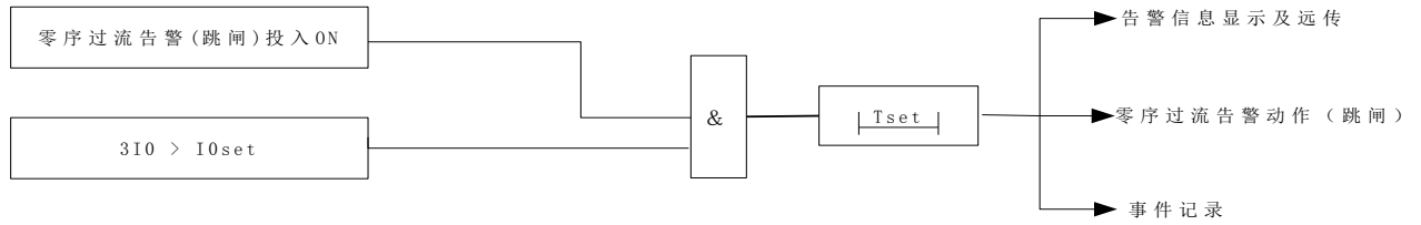
图 14 零序电流保护的逻辑图
