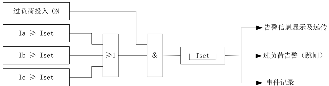
图 15 过负荷逻辑图
