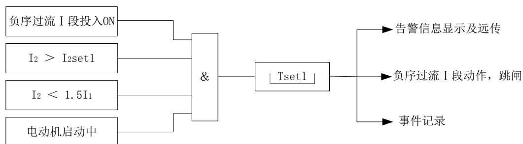
图 13 负序过流 I 段逻辑图
