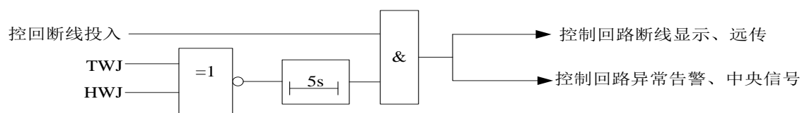
图 20 控制回路断线逻辑图
