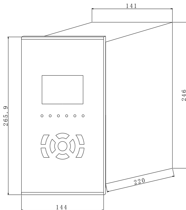
图1 NZB7173系列产品外形尺寸图
