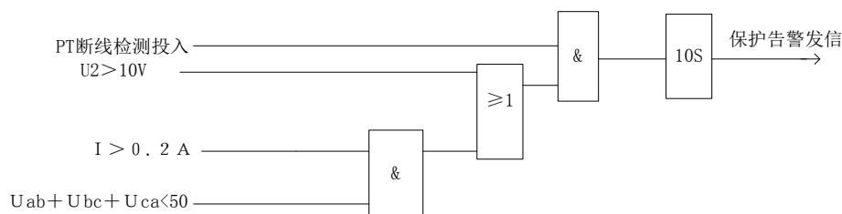
图 19 TV 断线逻辑图
