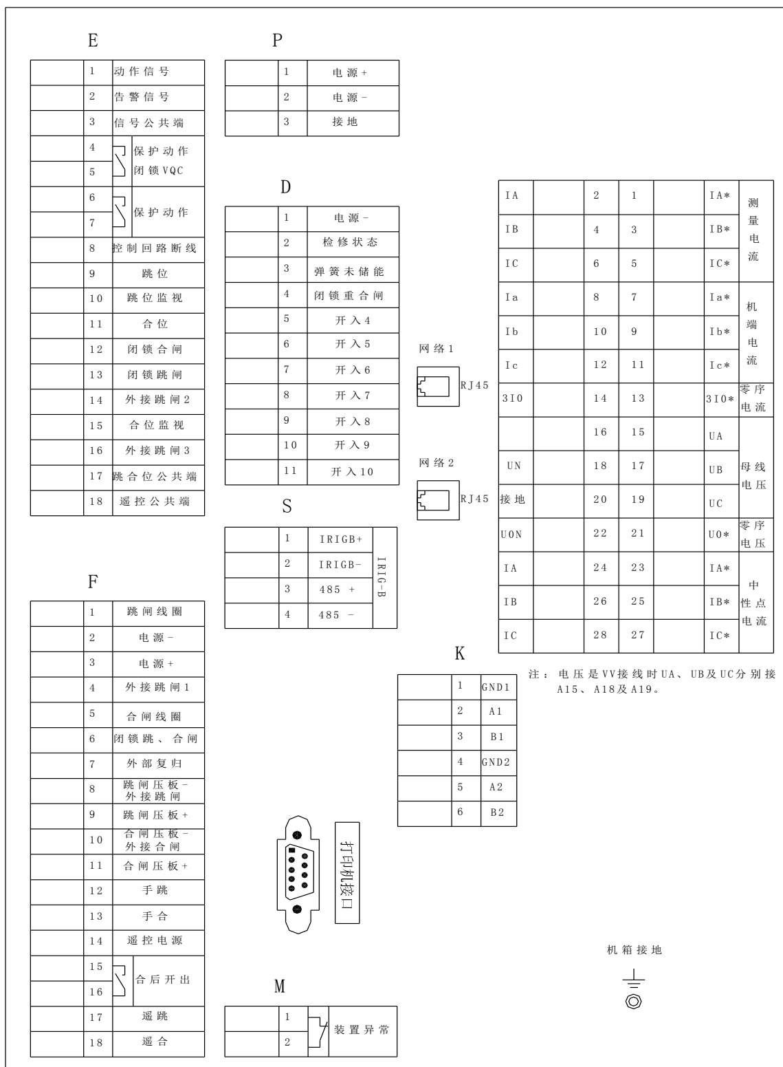
图 3 NZB7173 端子图
