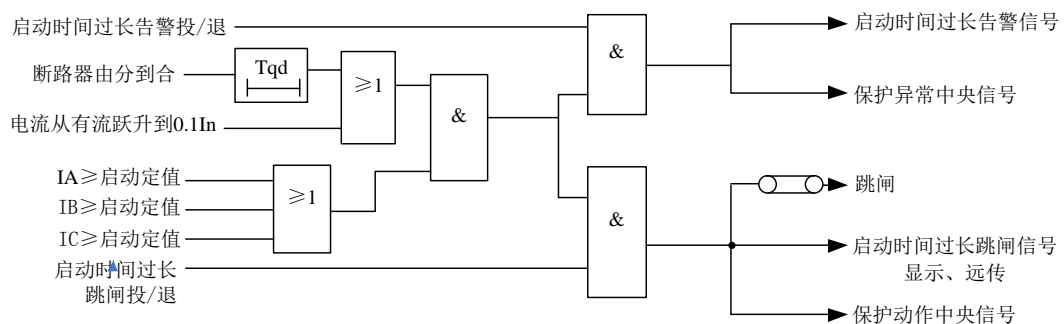
图 9 启动时间过长保护逻辑图
