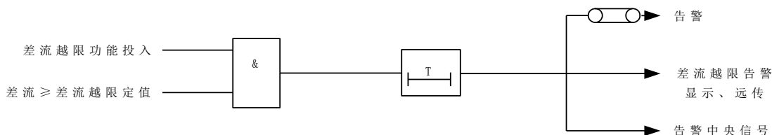
图 7 差流越限逻辑图
