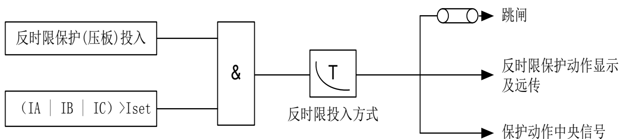
图 4 反时限保护逻辑图
