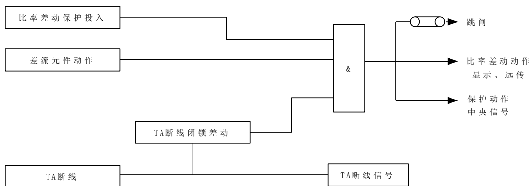
图 6 比率制动差动保护逻辑图
