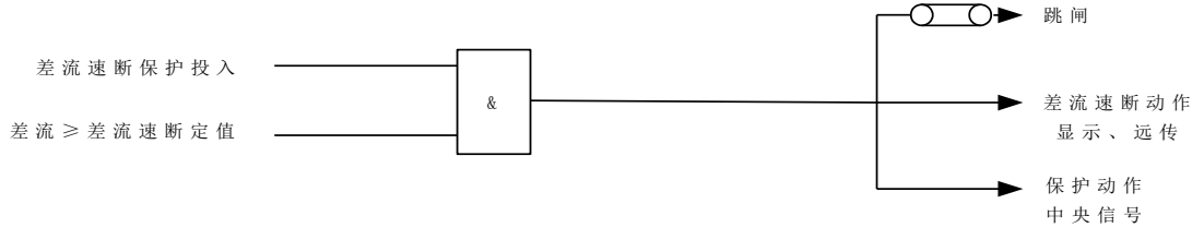
图 4 差流速断保护逻辑图
