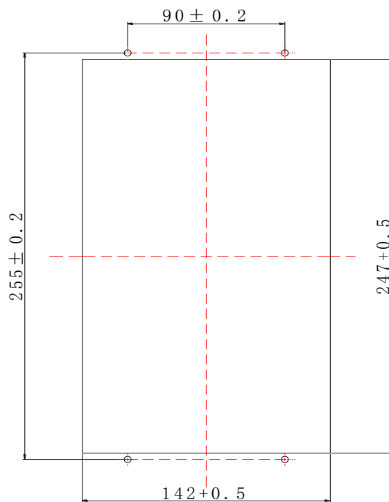
图2 NZB7173系列产品开孔尺寸图
