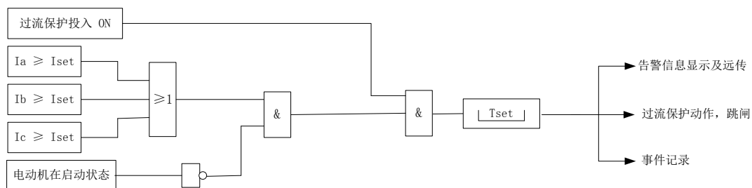
图 12 堵转保护逻辑框图
