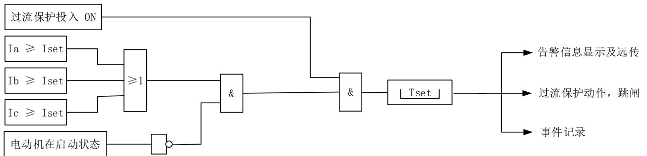
图 11 过流保护逻辑框图
