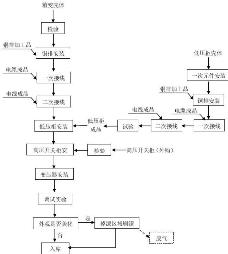
图 3-2 生产工艺流程
