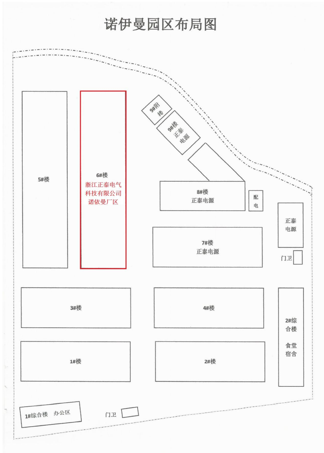
图 3-4 诺依曼厂区平面图
