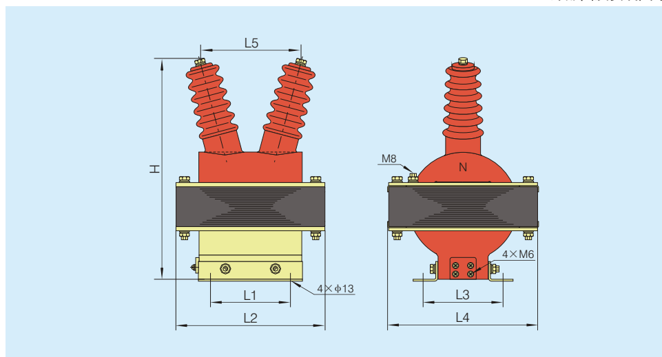
JDZJ-3、6、10外形图及安装尺寸
