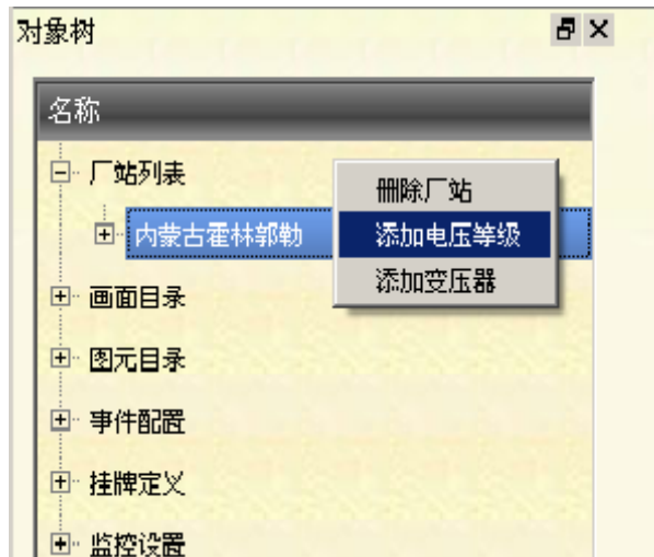
图 46 一次设备建模
