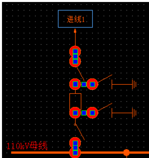
图 63 画面编辑区
