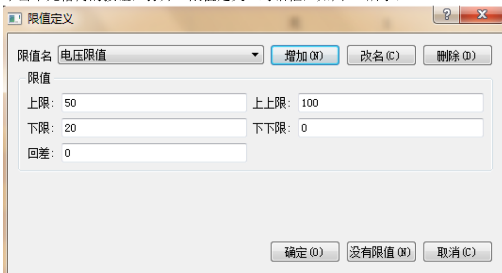
图 33 限值定义
