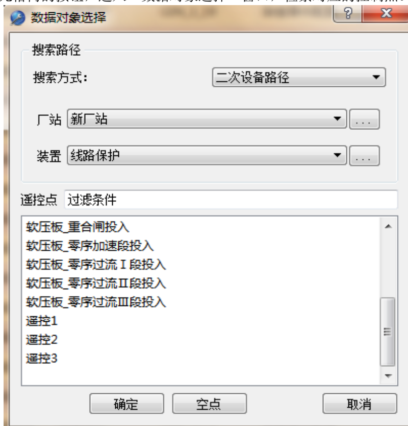
图 38 遥控点设置
