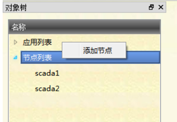
图 24 节点添加
