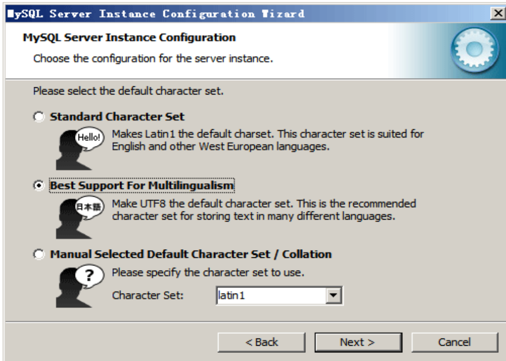
图 10 字符集选择
