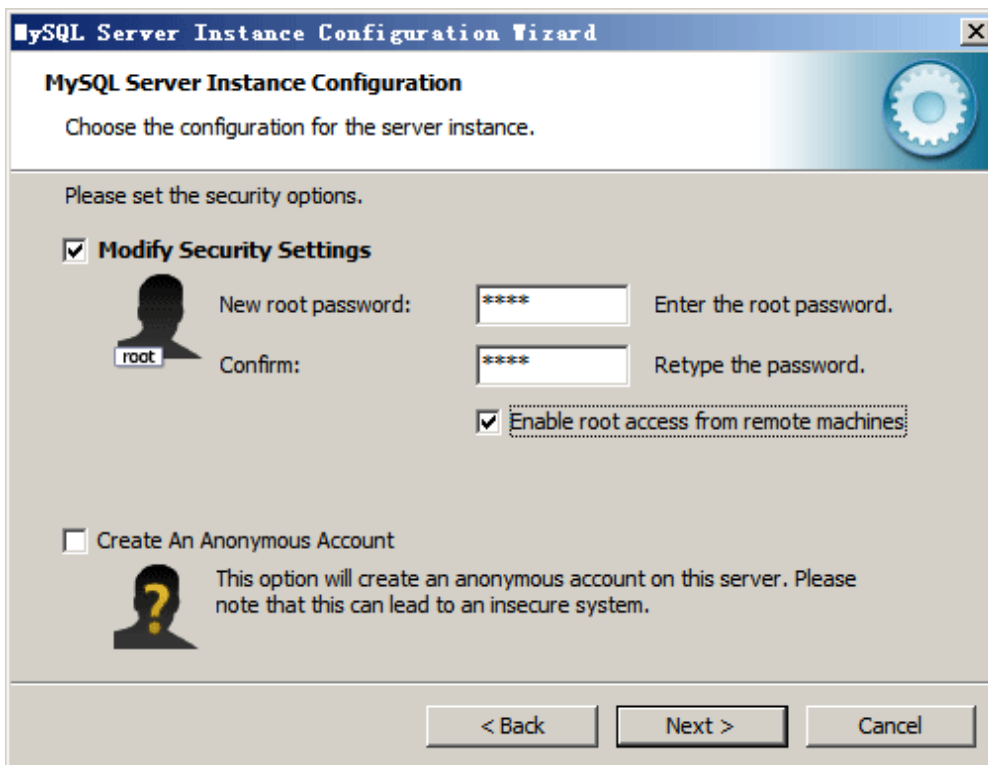
图 12 安全选项
