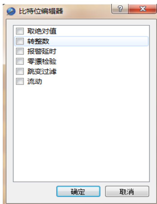
图 35 标记处理
