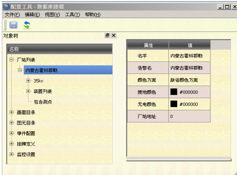
图 25 场站建模
