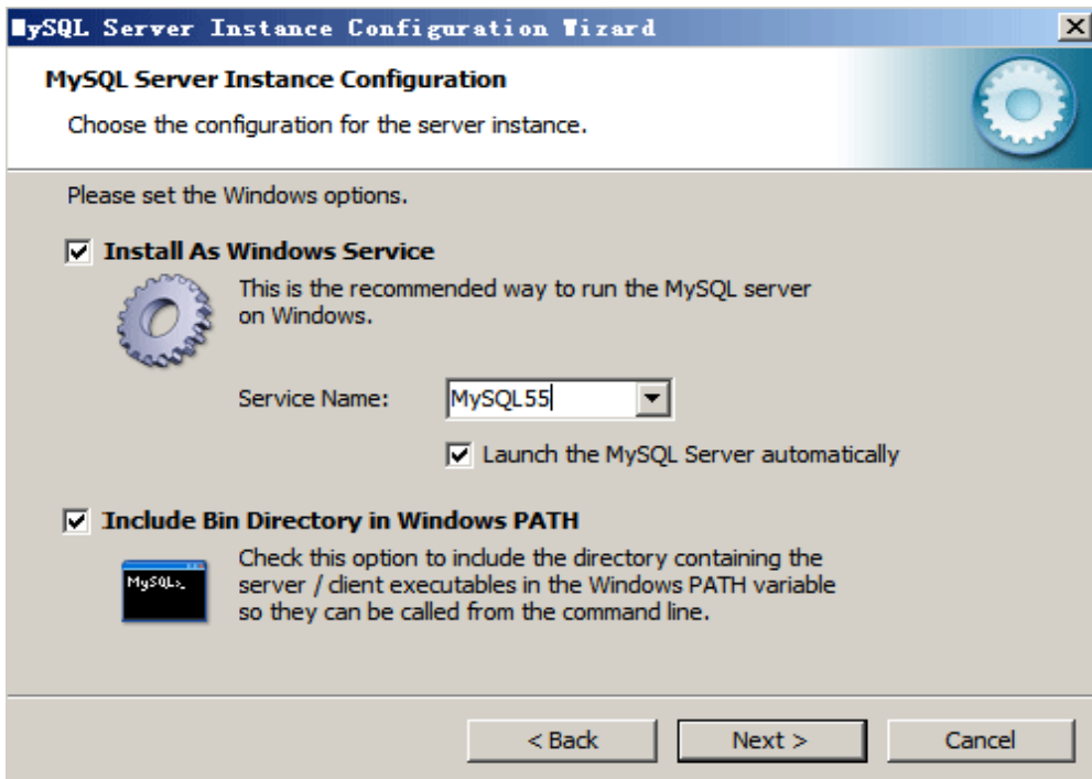
图 11 服务设置
