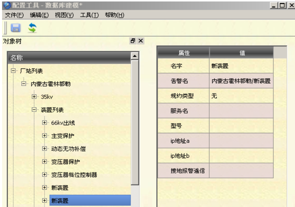
图 26 装置添加
