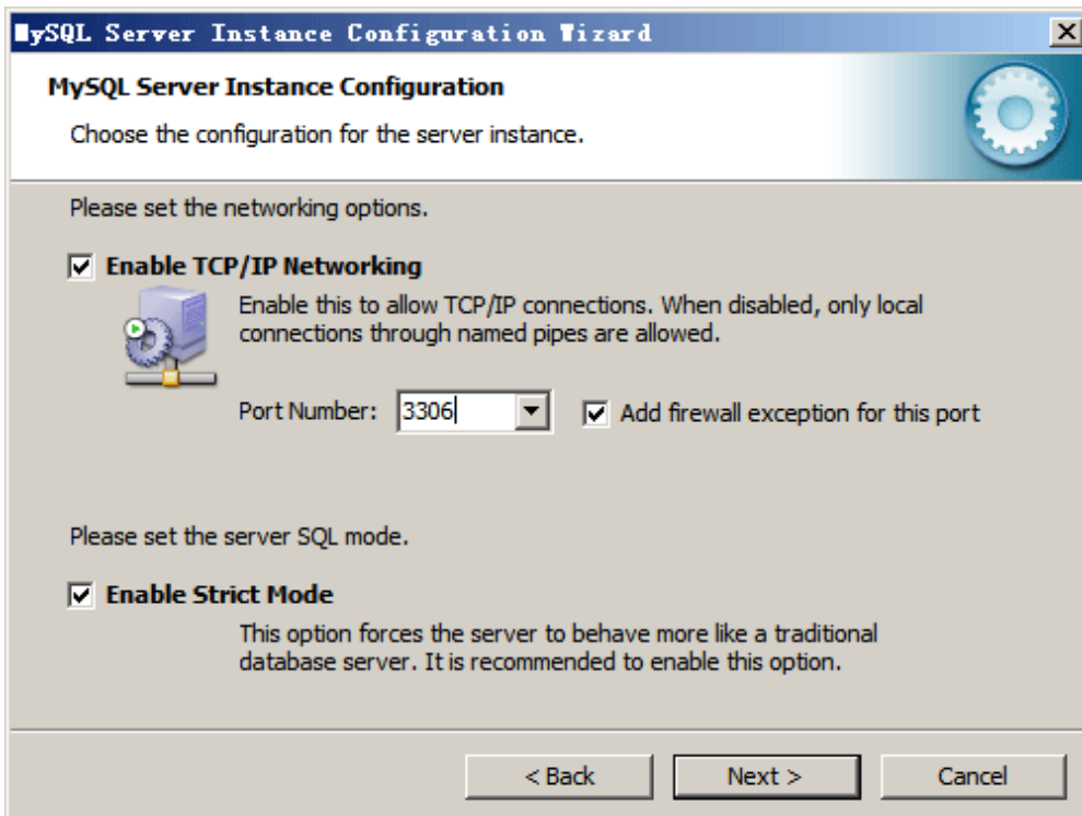
图 9 联网选择
