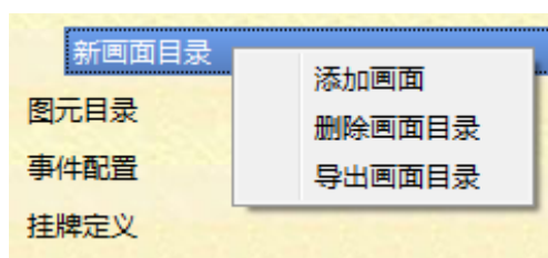
图 56 画面添加
