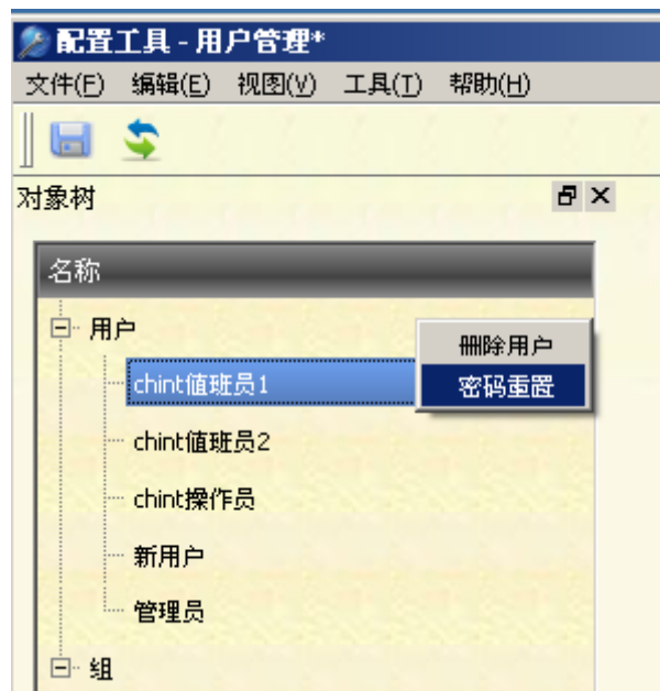
图 19 密码重置
