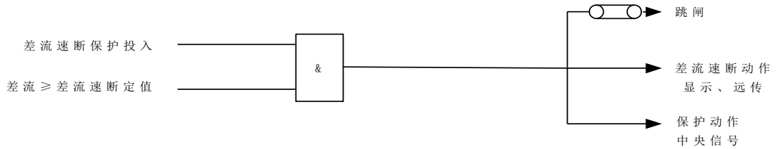
图 4 差流速断保护逻辑图
