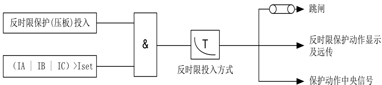
图 4 反时限保护逻辑图
