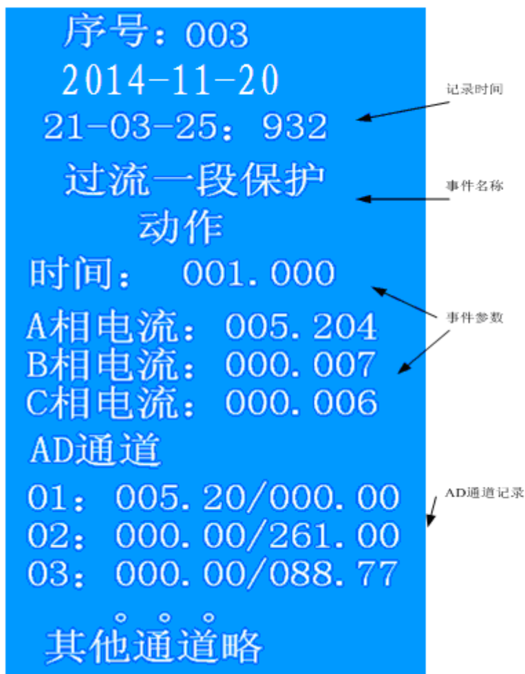
图 21: 事件记录
