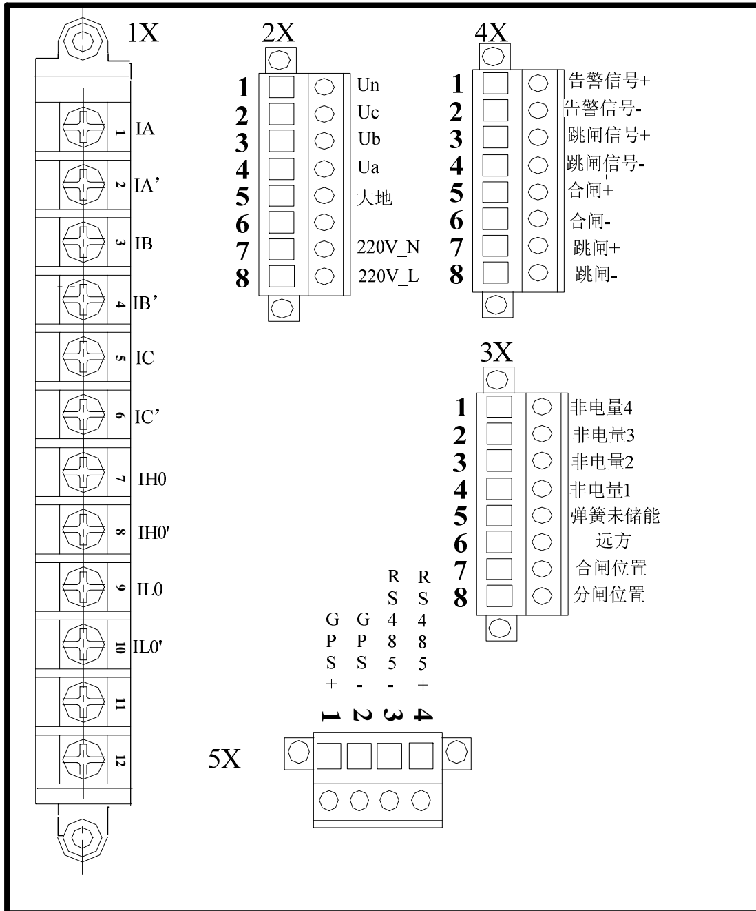
图 3: NZB6011 端子定义
