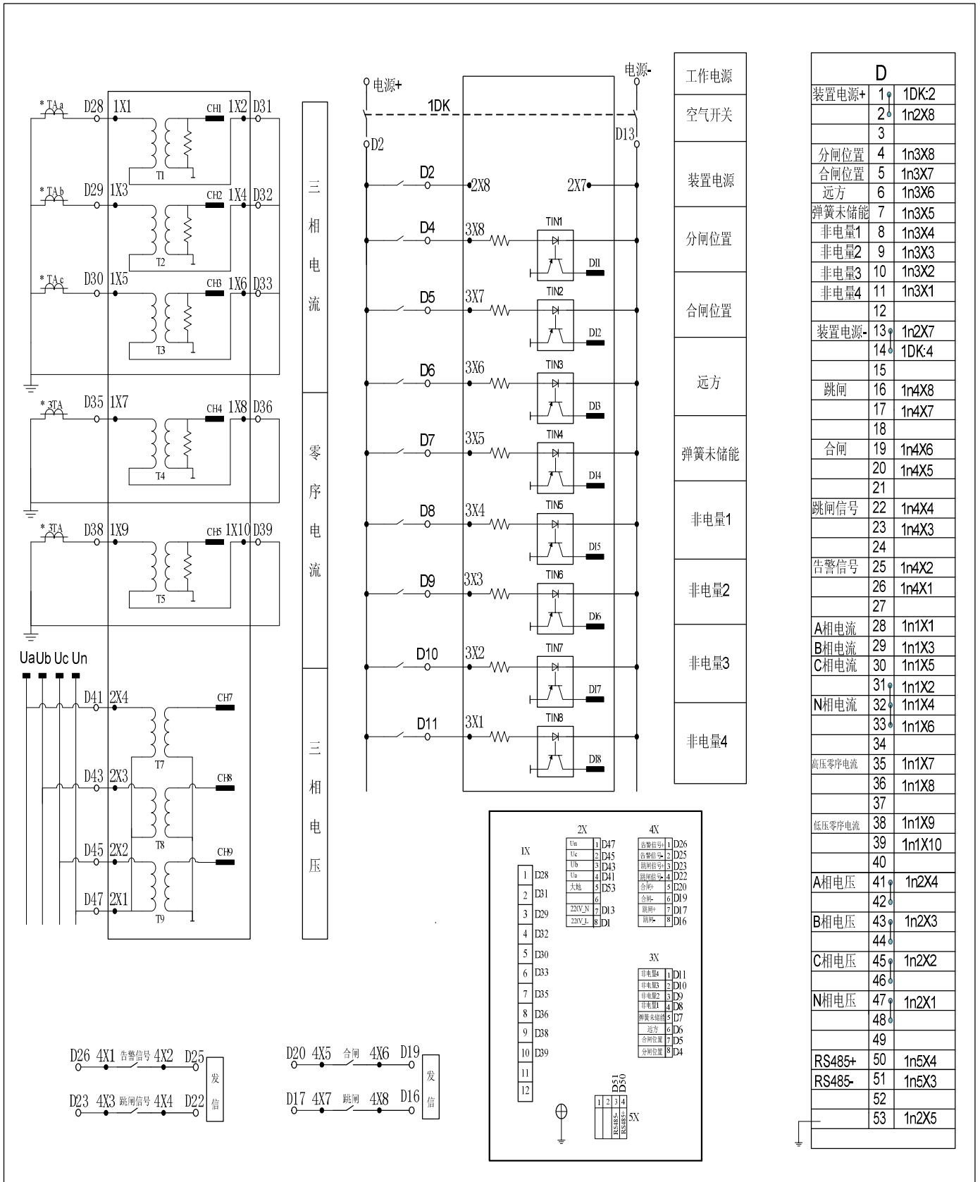
图 27 : NZB6011 典型接线图
