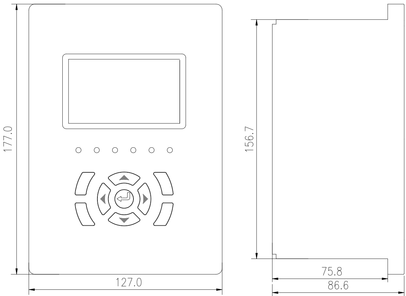
图 1: NZB6011 外形尺寸
