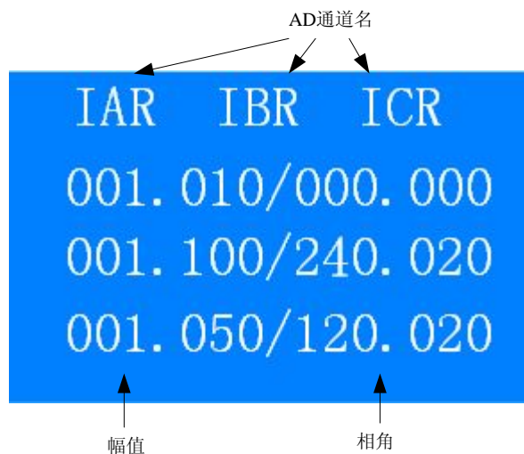
图 7: 基波显示
