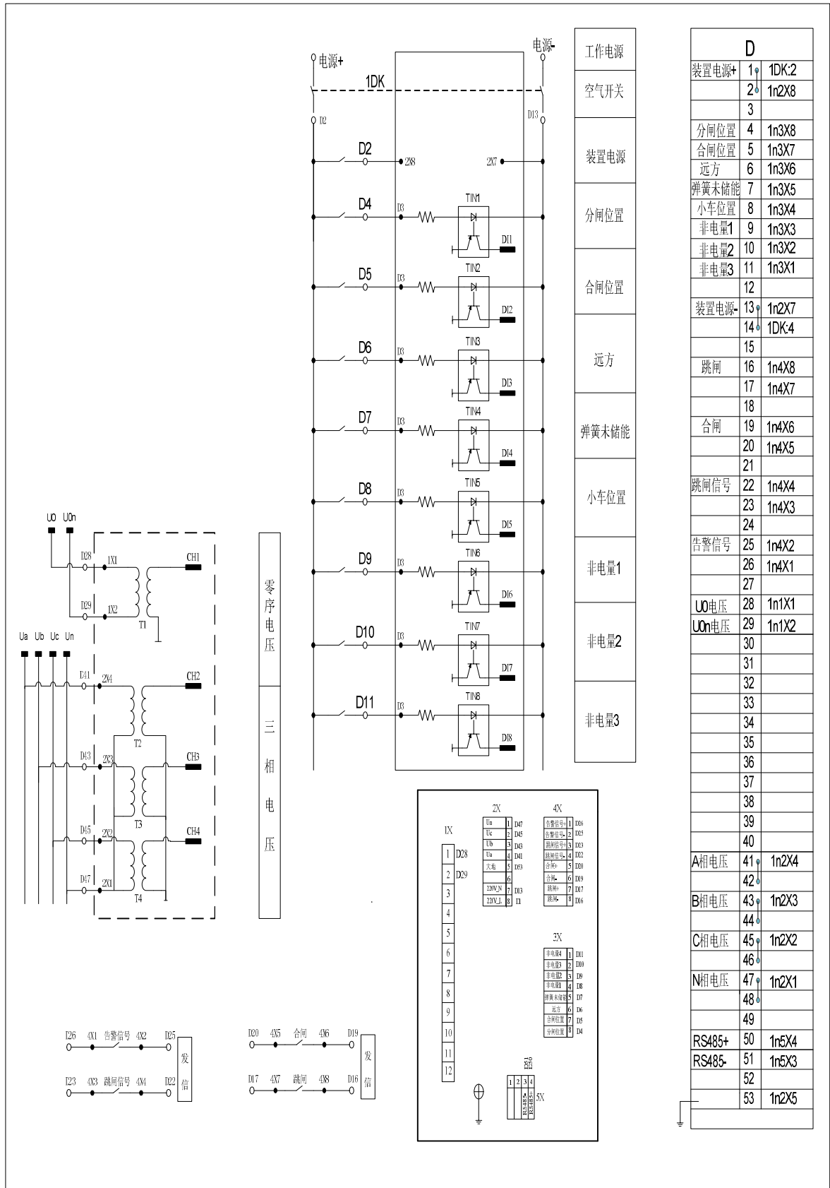
图 26 NZB6001 典型接线图
