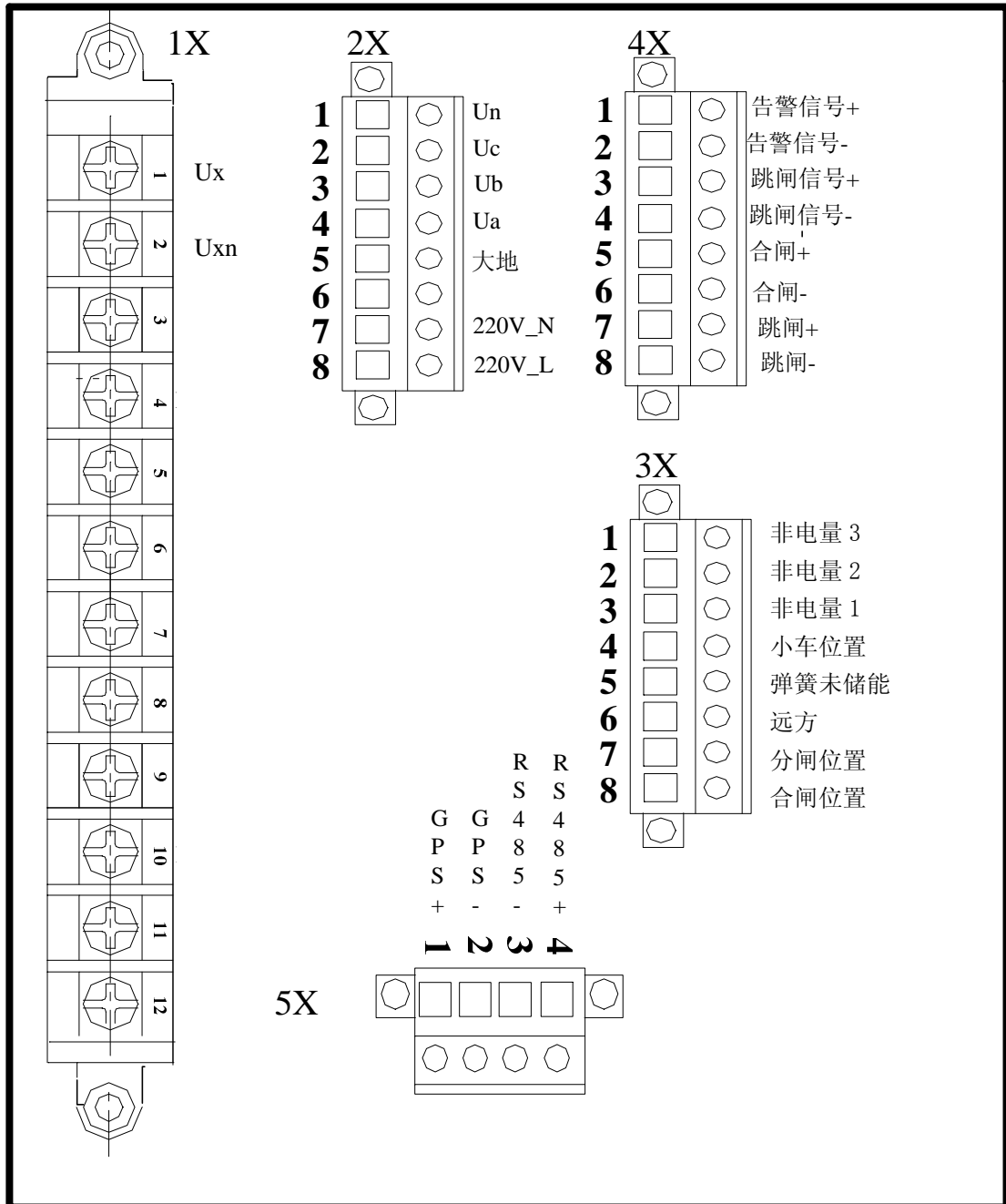
图 2: NZB6001 端子定义图
