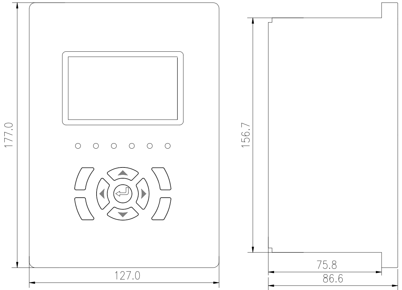
图 1: NZB6001 装置外形尺寸
