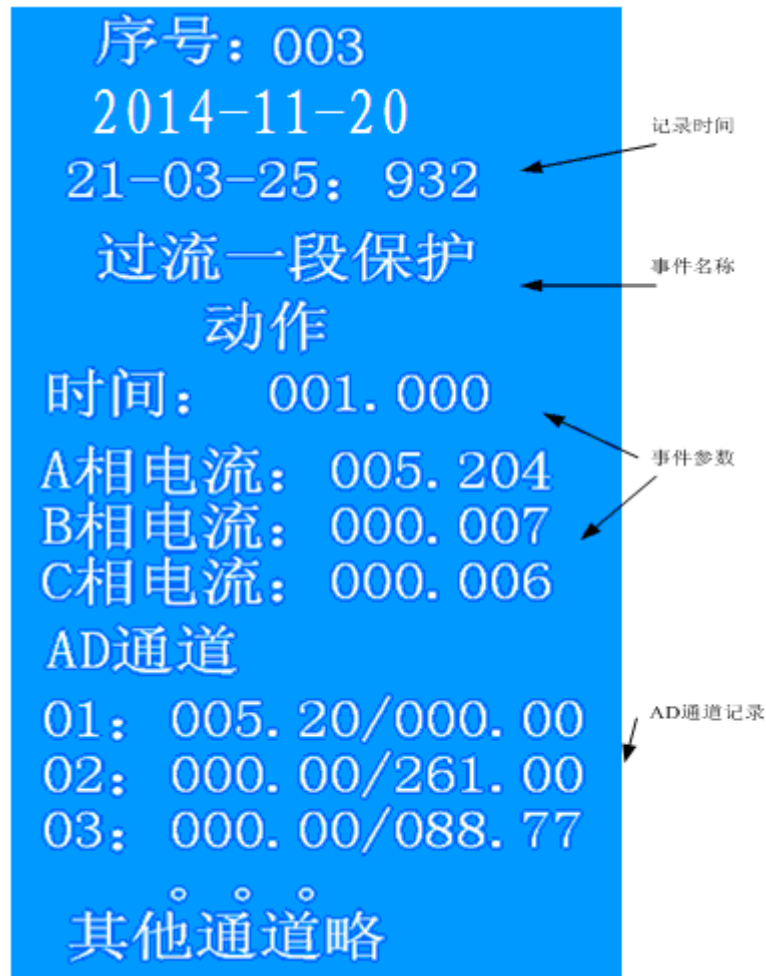
图 20: 事件记录显示界面
